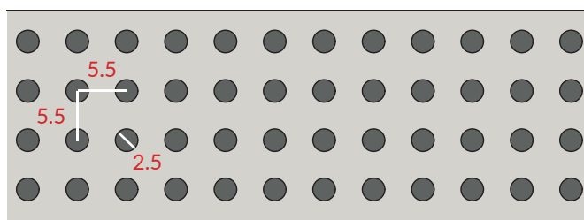
superficie perforata
