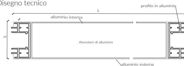
Disegno tecnico
