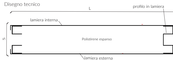
Disegno tecnico
